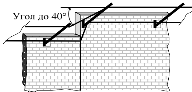
Рисунок 2.3 – Крепление КМЧ и проводов при перепадах высоты
