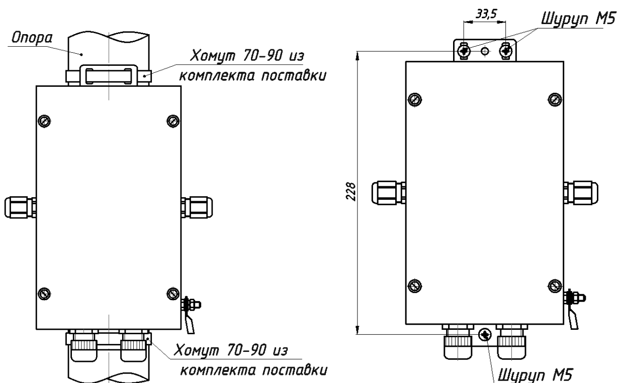
Рисунок 2 – Крепление коробки распределительной «БАРЬЕР-КР-В» ФРСБ.468344.004 на опоре
