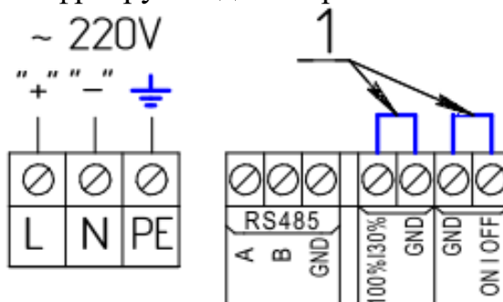
Рисунок 2.3 – Непосредственное подключение прожектора к сети электропитания
