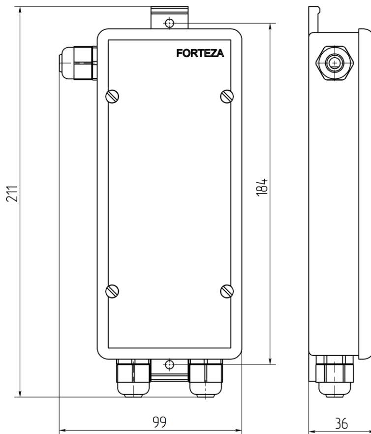
Рисунок 1 – Внешний вид коробки распределительной БАРЬЕР-КР-М ФРСБ.468344.001
