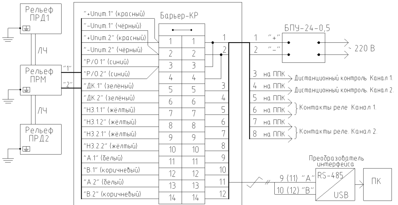
Рисунок 2.8 – Подключение извещателя к коробке распределительной (индикатор включен).
