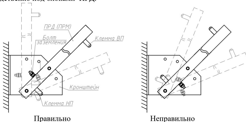
Рисунок 2.6 – Установка ПРД
