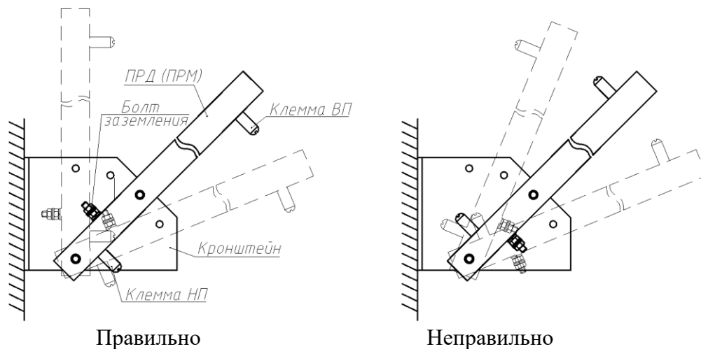
Рисунок 2.6 – Установка ПРД
