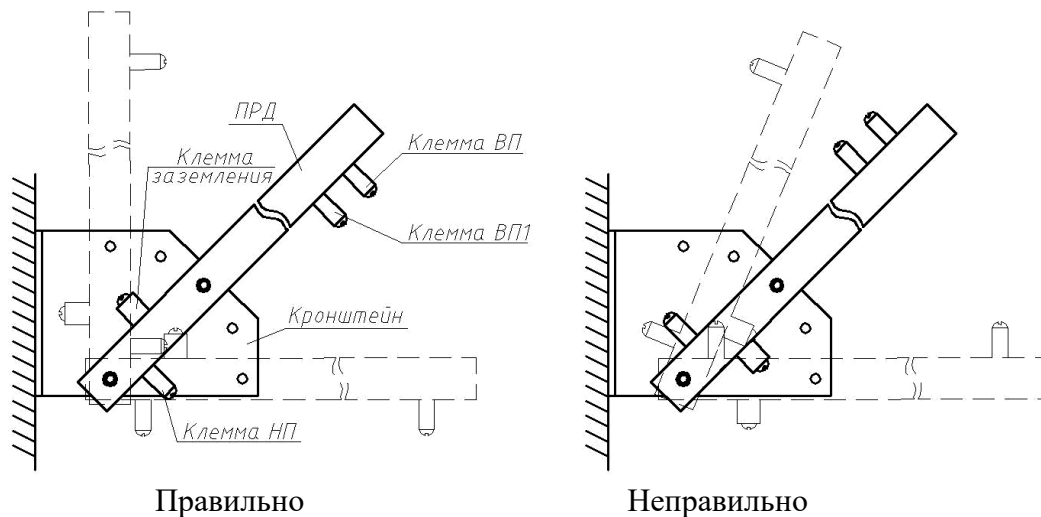
Рисунок 2.6 Установка ПРД
