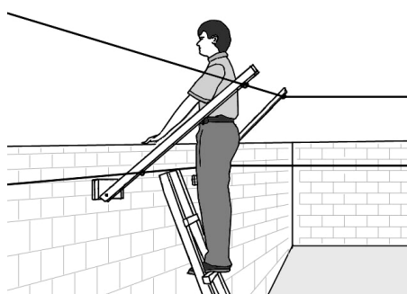
Рисунок 2.11. Имитация преодоления зоны обнаружения при козырьковом варианте установки.
