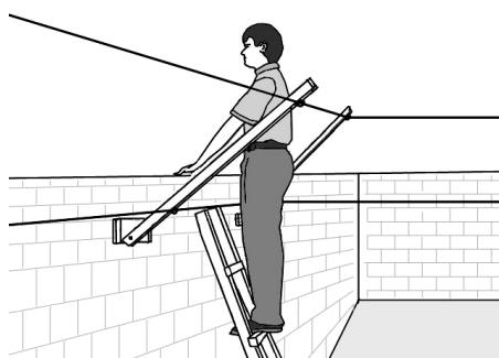
Рисунок 2.11. Имитация преодоления зоны обнаружения при козырьковом варианте установки.
