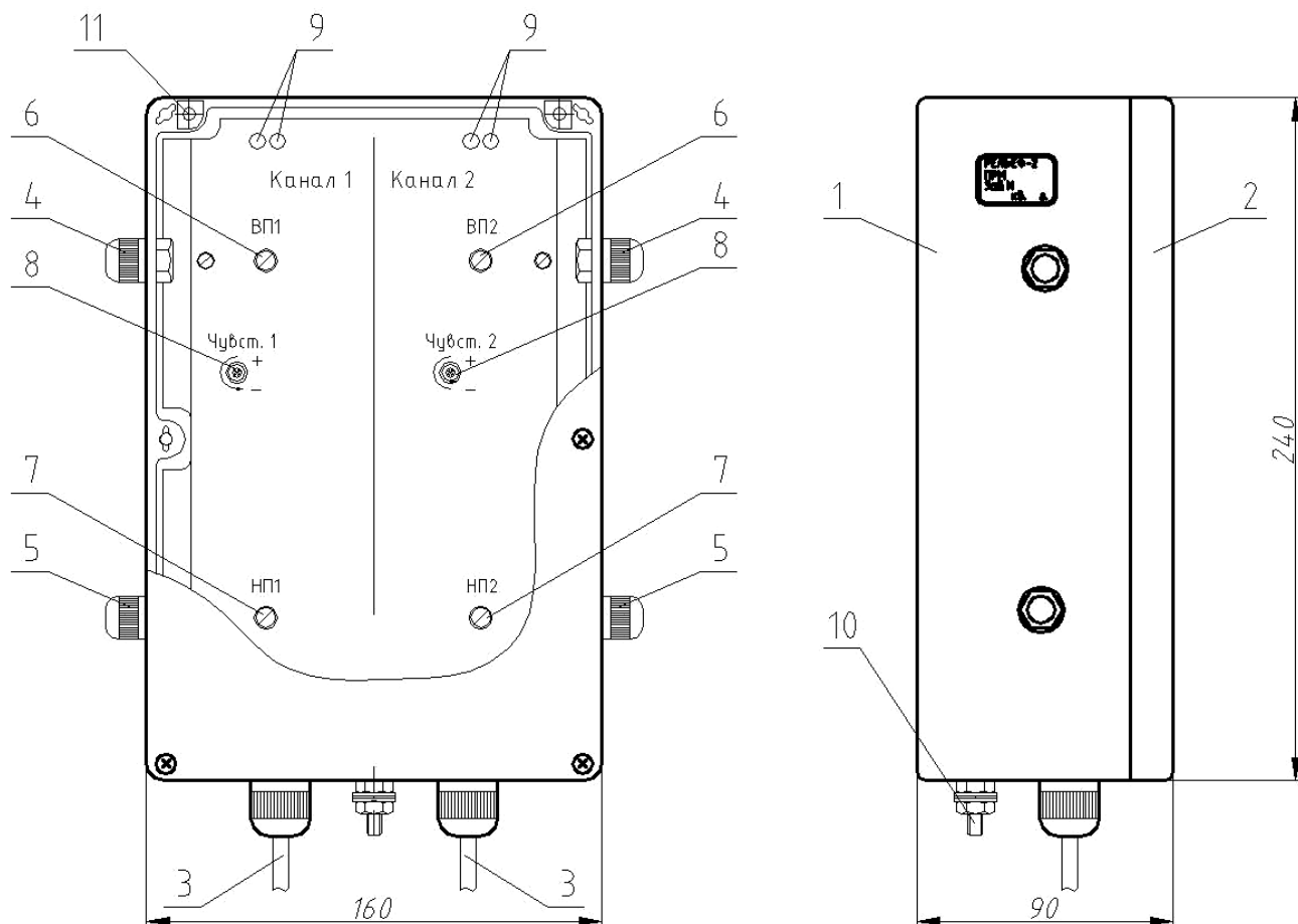
1 – корпус; 2 – крышка; 3 – выходные кабели; 4 – кабельные вводы для ВП ЛЧ; 5 – кабельные вводы для НП ЛЧ; 6 – клеммы ВП1, ВП2; 7 – клеммы НП1, НП2; 8 – регуляторы чувствительности; 9 – двухцветные индикаторы; 10 – клемма заземления; 11 – отверстия для крепления блока на стену.
