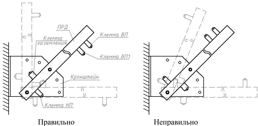
Рисунок 2.6 Установка ПРД
