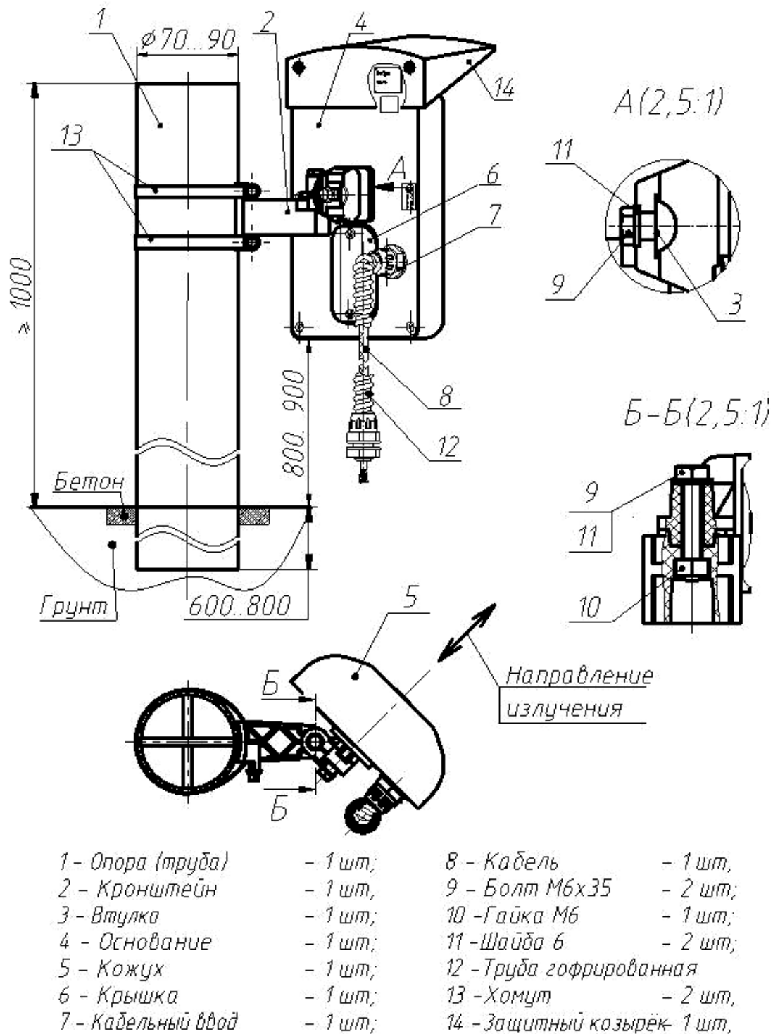
Рисунок 6.1 Установка извещателя на опоре
