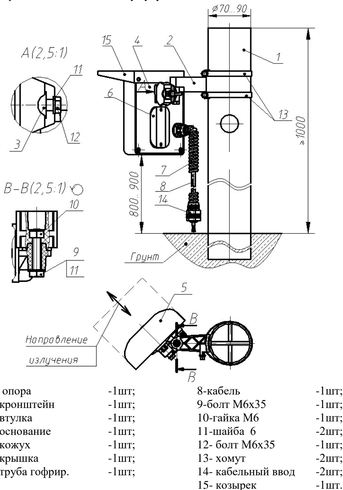
Рисунок 6.1 Установка извещателя на опоре
