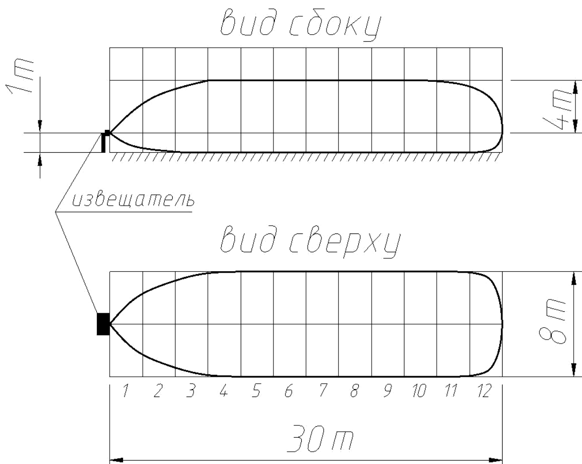
Рисунок 8.1 Зона обнаружения извещателя при установке на участке периметра на высоте 1 метр.
