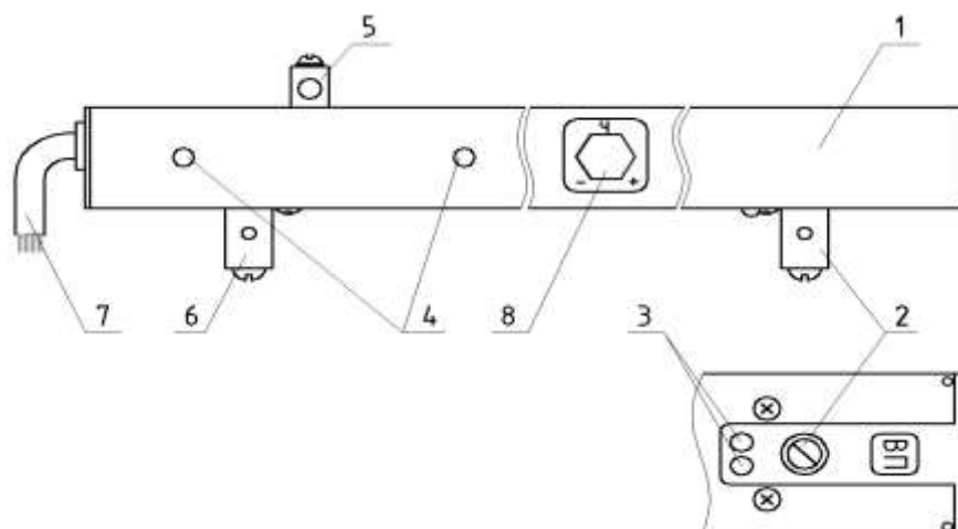
Рисунок 1.3 Конструкция ПРМ.
