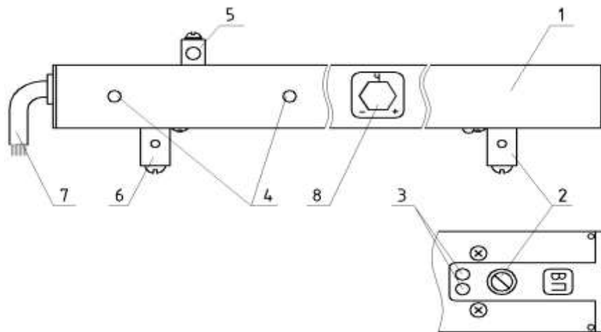
Рисунок 1.3 Конструкция ПРМ.
