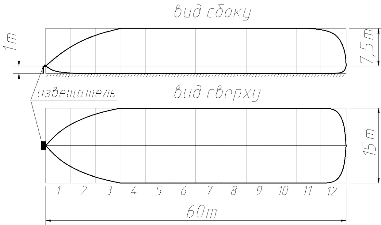
Рисунок 8.1 Форма и размеры зоны обнаружения извещателя для варианта исполнения «объем» при установке на высоте 1 метр.
