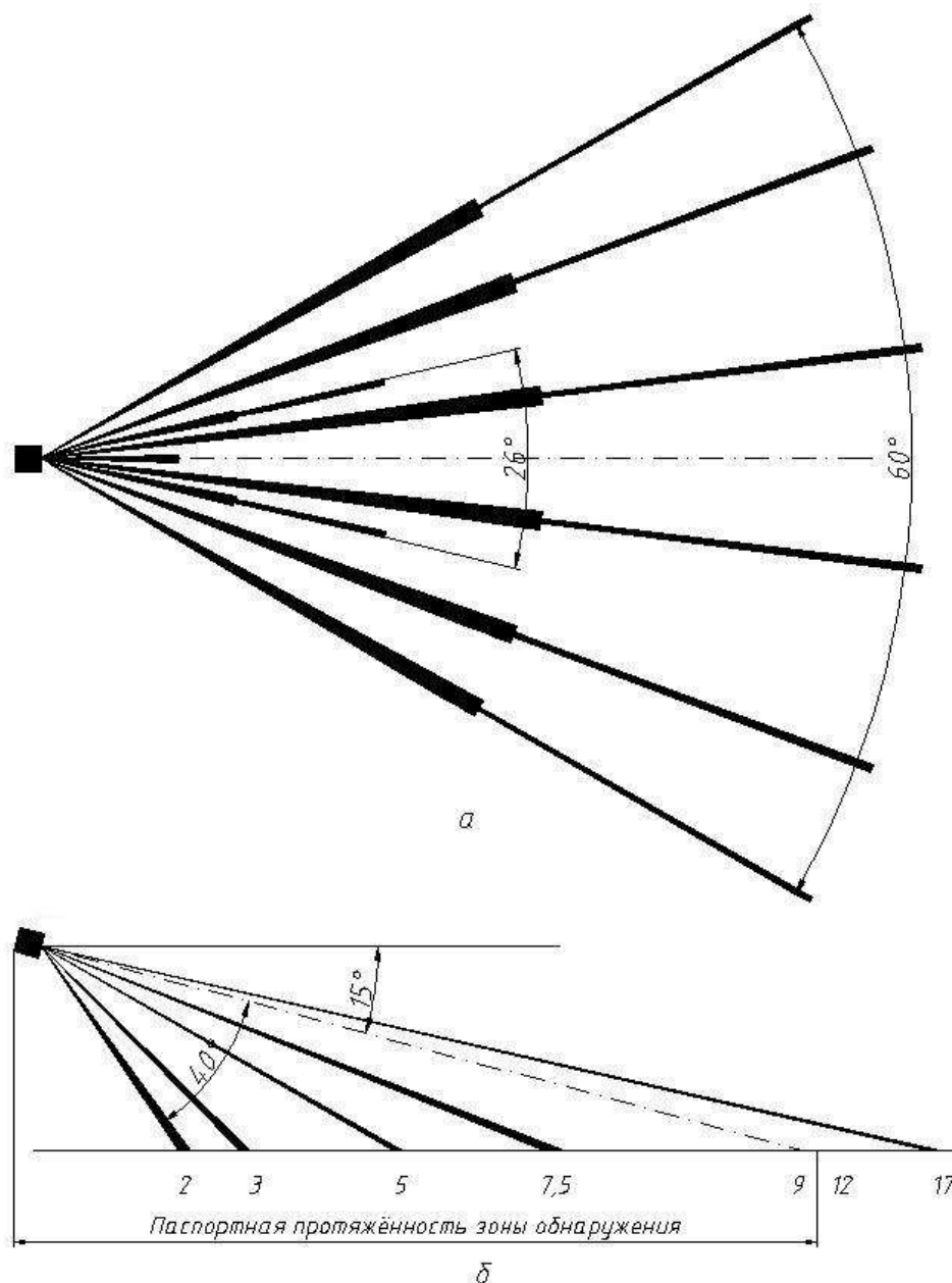
Рисунок 3.1 Диаграмма направленности зоны обнаружения при установке на высоте 2,5...3 м.
